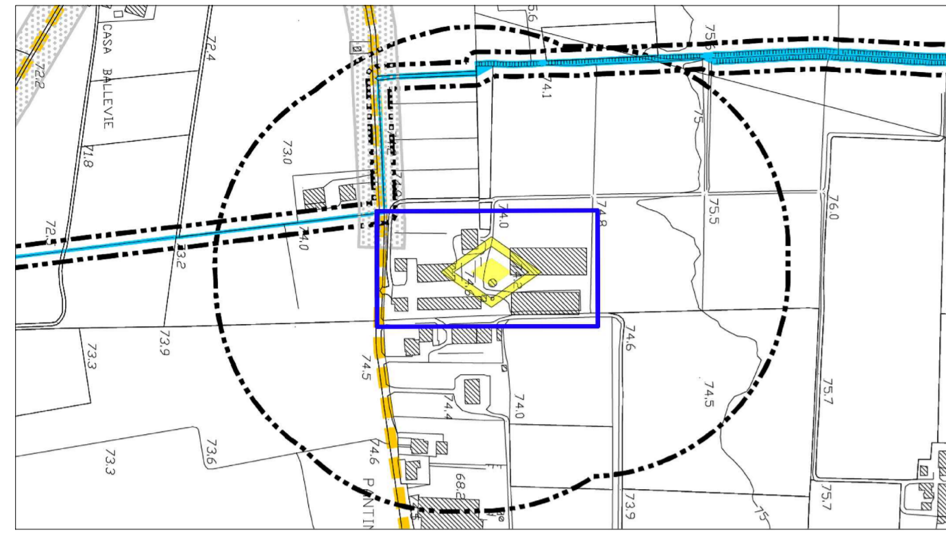
STRALCIO P.A.T. - TAVOLA 1 "ALLEVAMENTI ZOOTECNICI INTENSIVI - FASCE DI RISPETTO"
