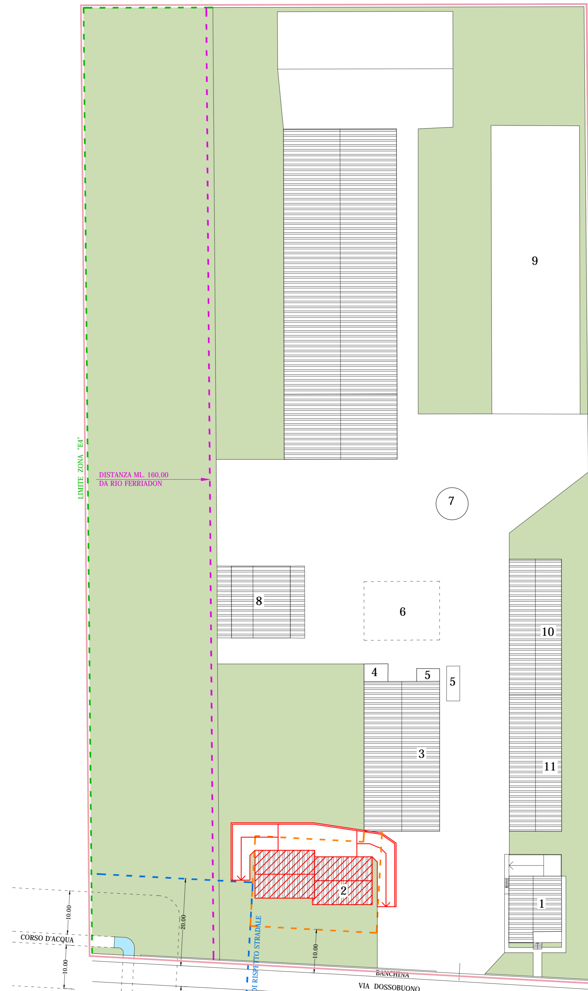
STATO DI VARIANTE PLANIMETRIA GENERALE SCALA 1:500
