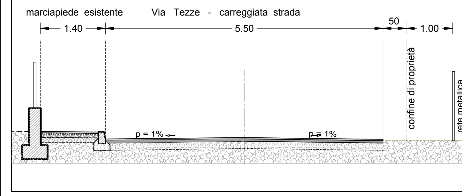
Sezione stradale stato Attuale sc. 1:50
